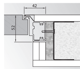
ellentétes éllel (befelé nyíló)
