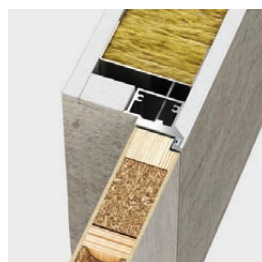
Fordított falc (befelé nyíló) - balos ajtó
